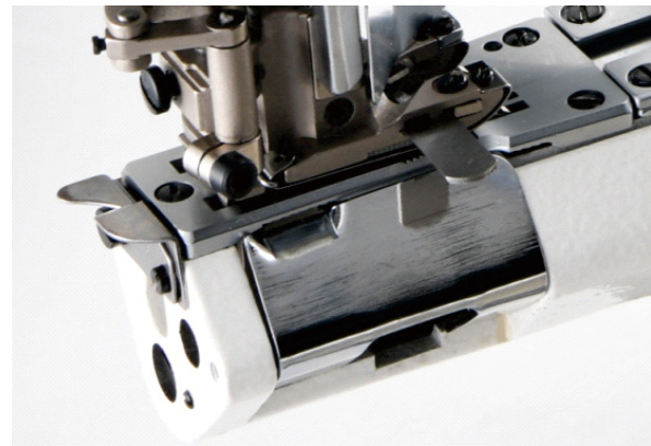
弹片式压脚结构，面料适应性广
