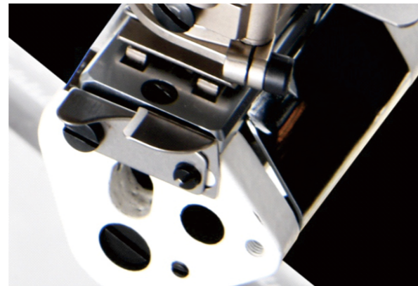
头部密封设计，无油污烦恼
